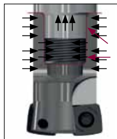
DUOPLUG® Schrumpf-/Schraubverbindung
